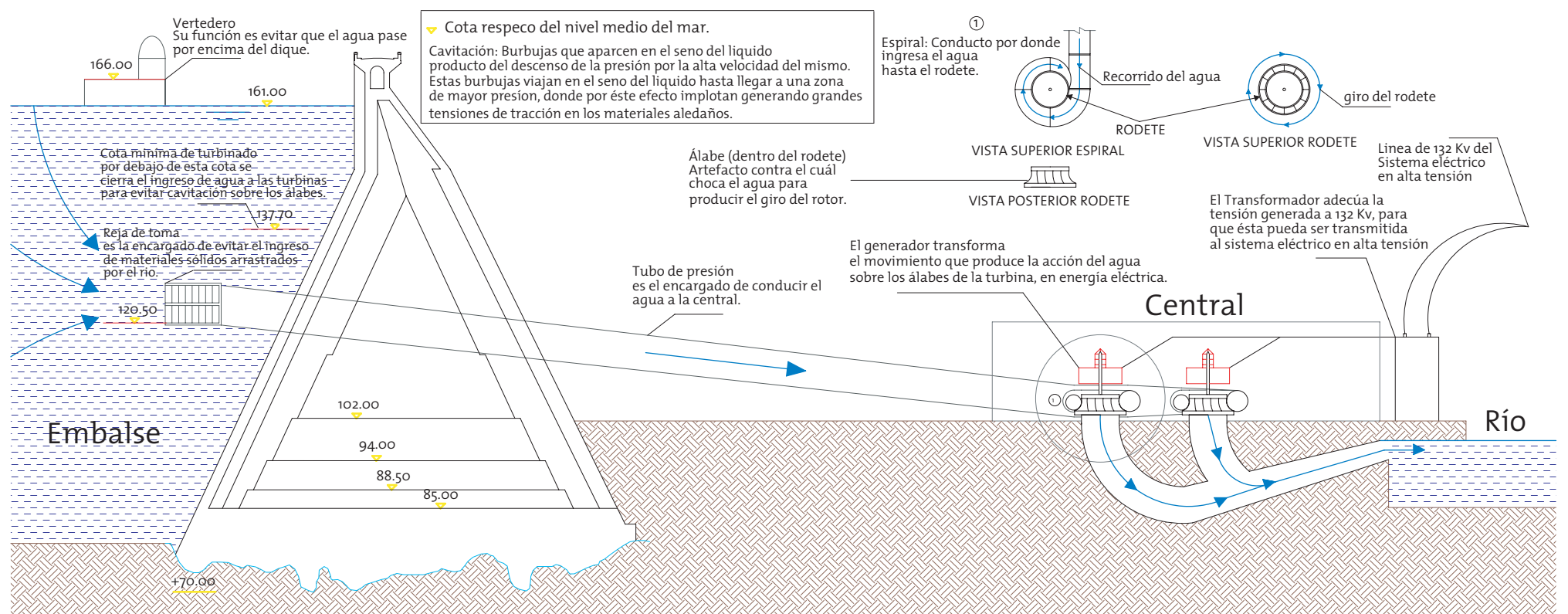
LA ALTURA GENERA QUE EL AGUA CAIGA CON VELOCIDAD HACIENDO GIRAR LAS TURBINAS
